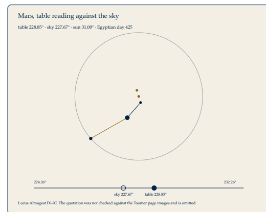
Figure 4 The same construction on Egyptian day 425. Table longitude 228.85°, sky longitude 227.67°.
