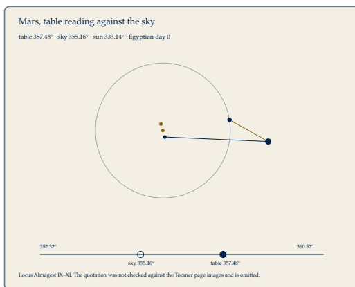
Figure 3 Mars on Egyptian day 0. Filled mark: Almagest longitude 357.48°. Open mark: DE441 longitude 355.16°.
